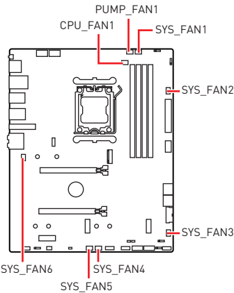
风扇接口规格
